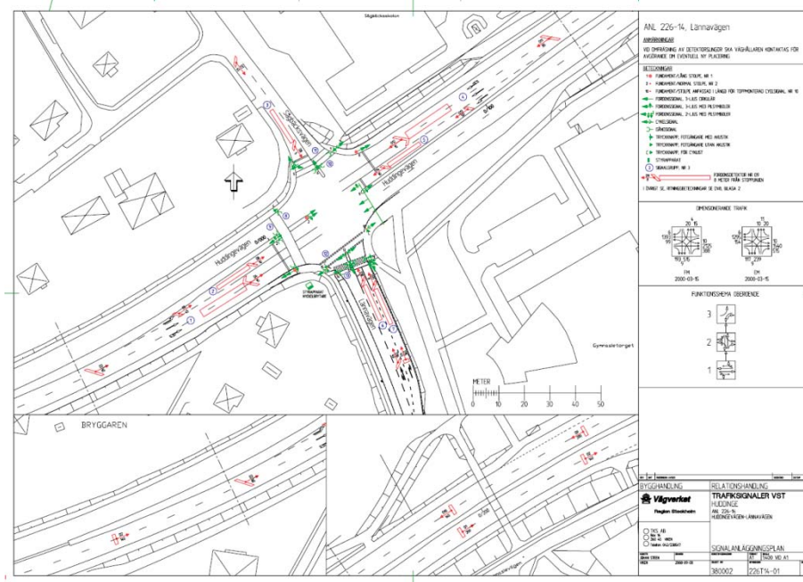
Figur 3 Exempel på signalanläggningsplan
