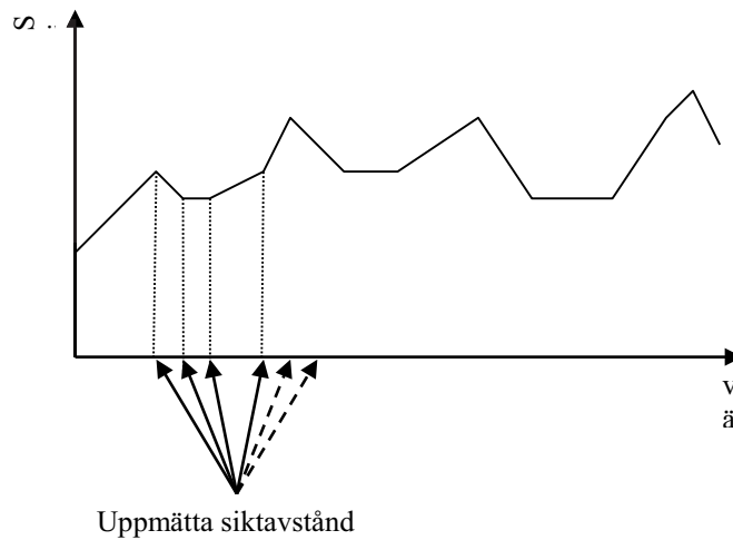
Figur 1 Exempel på siktavståndsprofil
